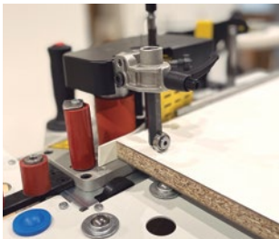
Palpador para el guiado del tablero.
