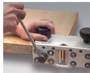
Sistema de corte con dos cuchillas. Equipado con cuchillas afilables de calidad profesional.
