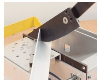
Extremo de la cuchilla biselado para el corte a medida de canalones en PVC
