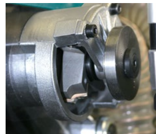
Copiador independiente de la fresa lo cual evita el marcado accidental del panel a perfilar.
