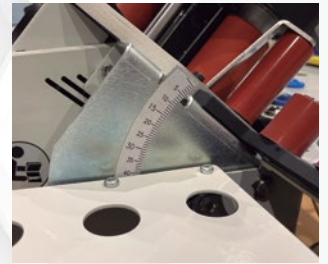
Inclinación de la máquina graduable hasta 45° para el aplacado de cantos biselados.
