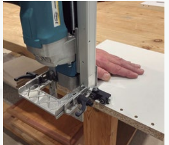
Multitaladro ref. 7946704 (incluido) Con tope de posicionamiento multitaladro paso 32. Ideal para la colocación de baldas intermedias móviles.
